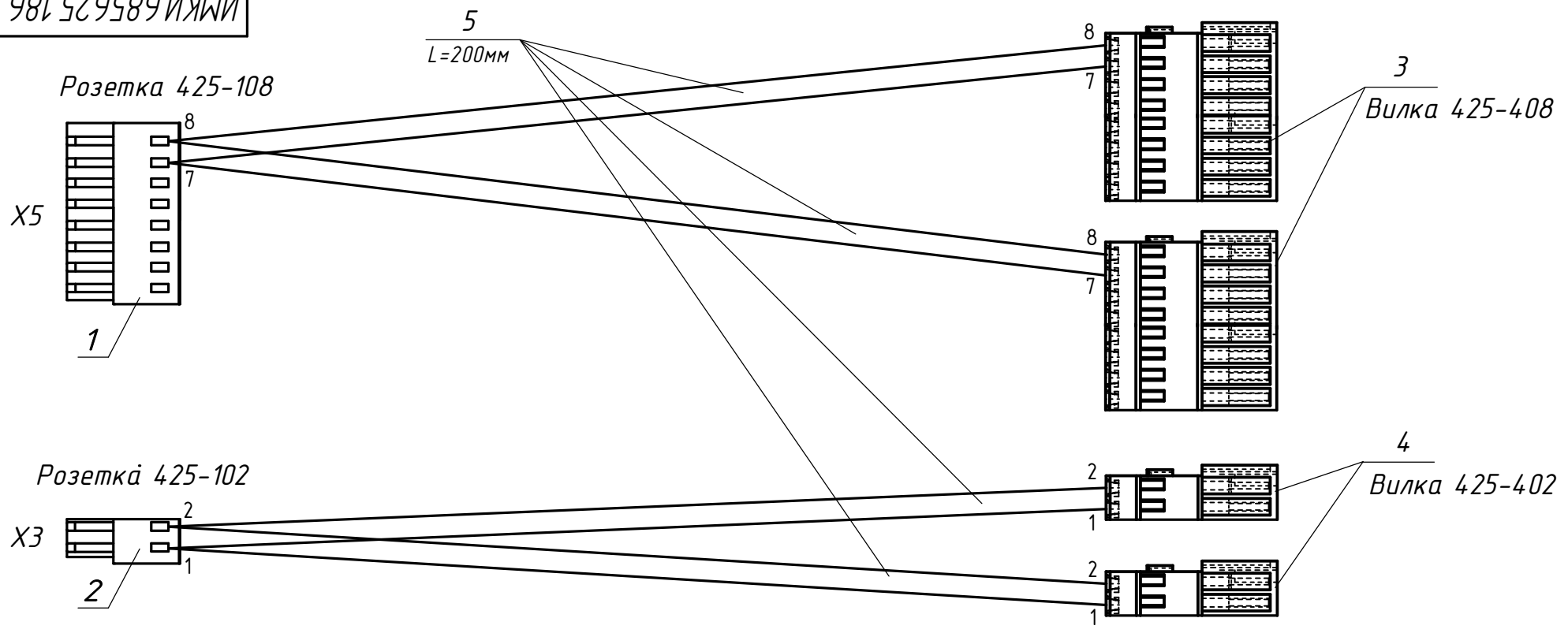
Розетка 425-108 (SUPU)
