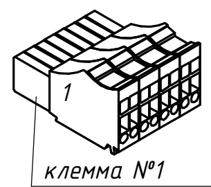
Розетка 2020-108 (WAGO)
