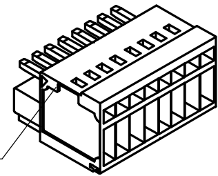
клемма №1
