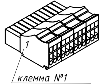
Розетка 2020-112 (WAGO)
