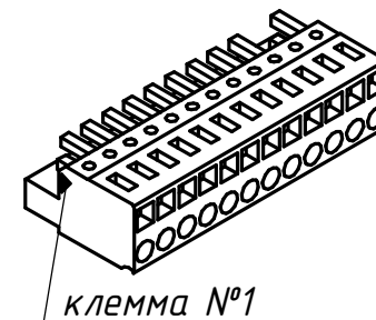
Розетка 450-112 (SUPU)
