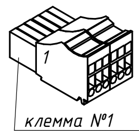
Розетка 2020-106 (WAGO)
